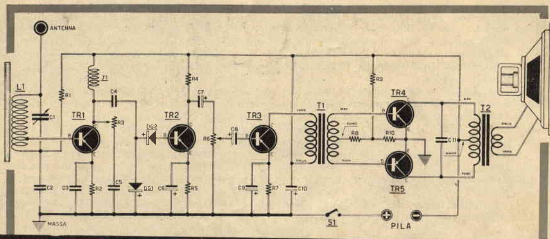
Fig. 1 - Schema elettrico del ricevitore Jaguaro.
