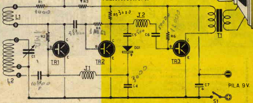
Fig. 1 - Schema elettrico del radoricevitore.
